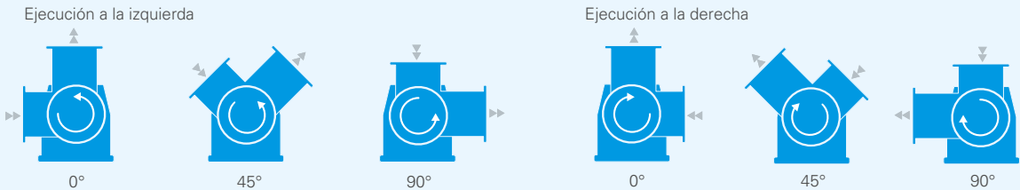
Variabilidad de las posiciones de las conexiones (sección A-A)
