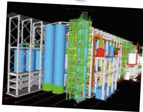
Nile Sugar Company / Ägypten: Komplette Planung der neuen Rübenzuckerfabrik – Konzept, Basic- und Detail-Engineering
