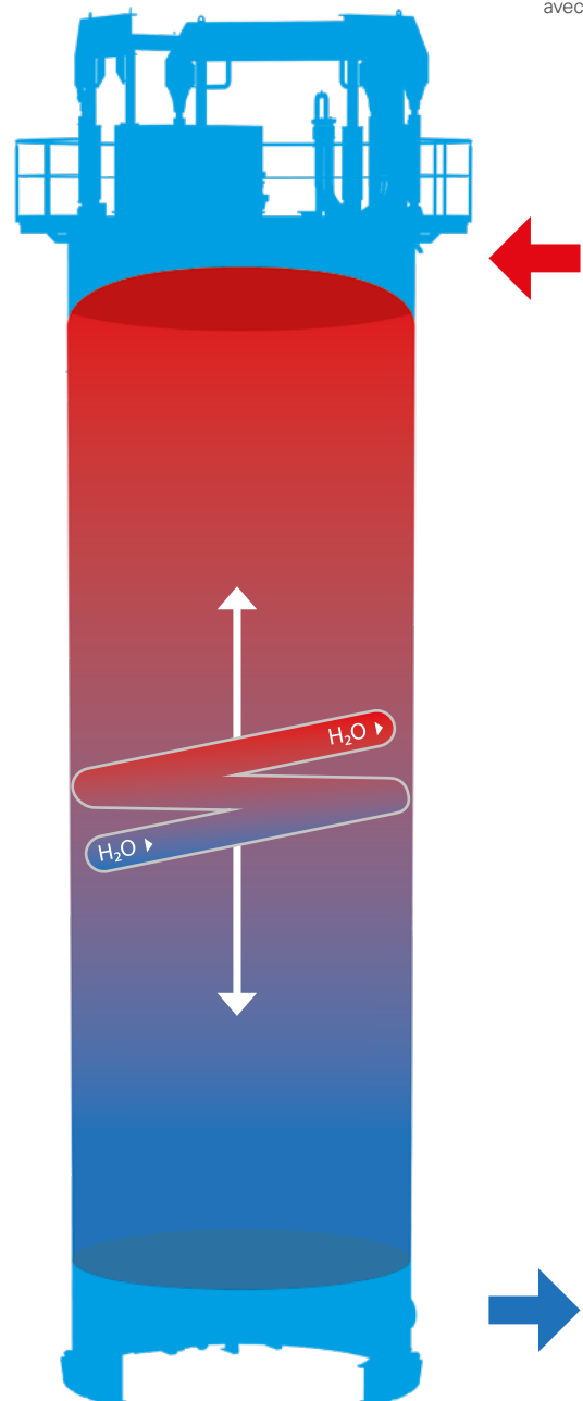
Schéma de la cristallisation par refroidissement
